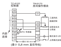
接线至带 NTC 传感器的 TM-9170 房间操作模块
