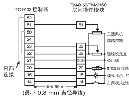
接线至 TM-9150/TM-9160 房间操作模块
