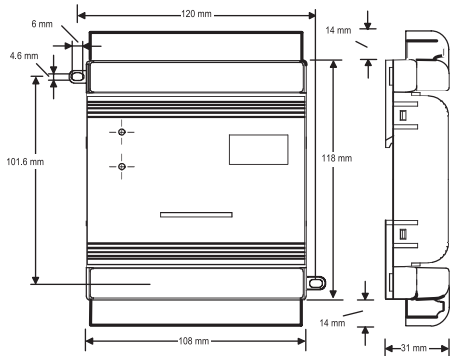
尺寸 (mm)
