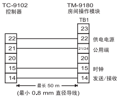
接线至 TM-9180 房间操作模块
